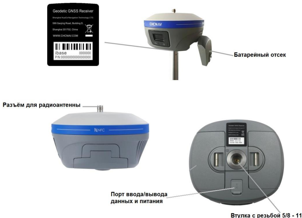
Рис.1.2. Корпус приёмника IBase
